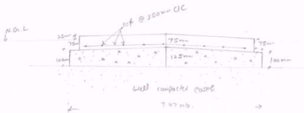
Section ①-①
