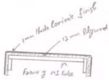
Section ①-①
